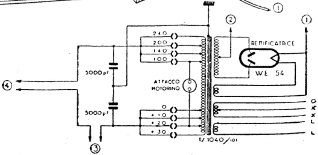
PHONOLA (S. A. FIMI). — Mod. «870». - Particolari del blocco di alimentazione.
